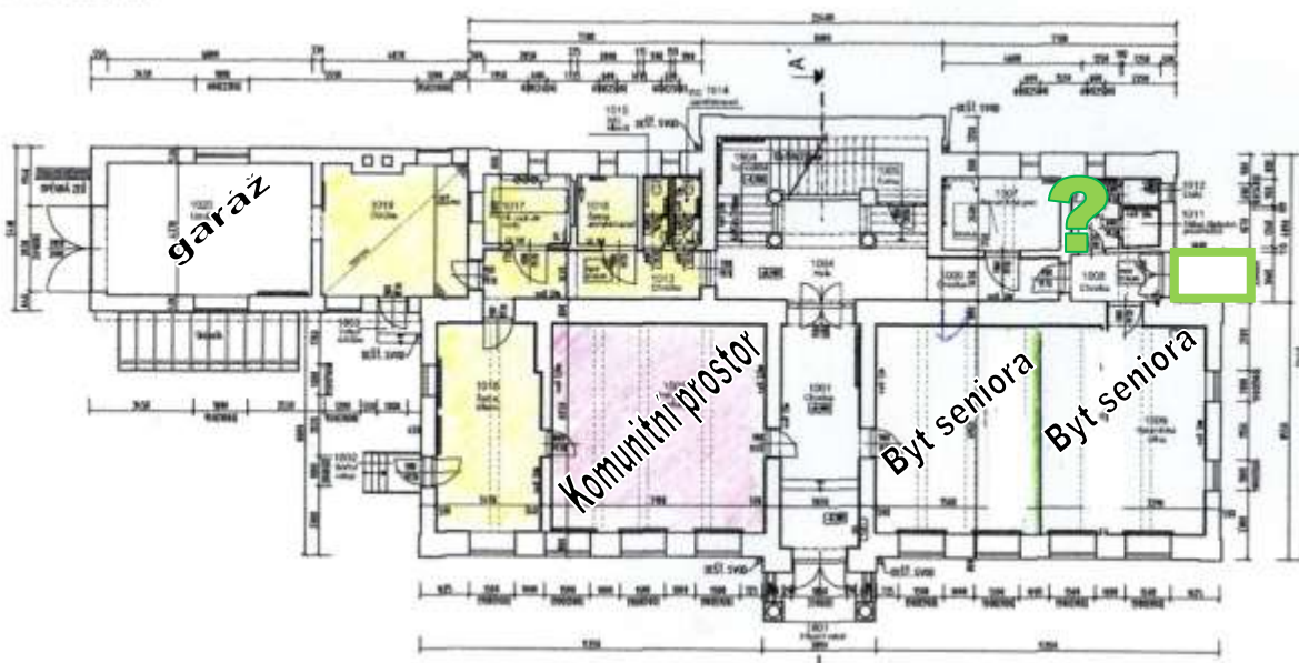
PŮDORYS 1.NP
